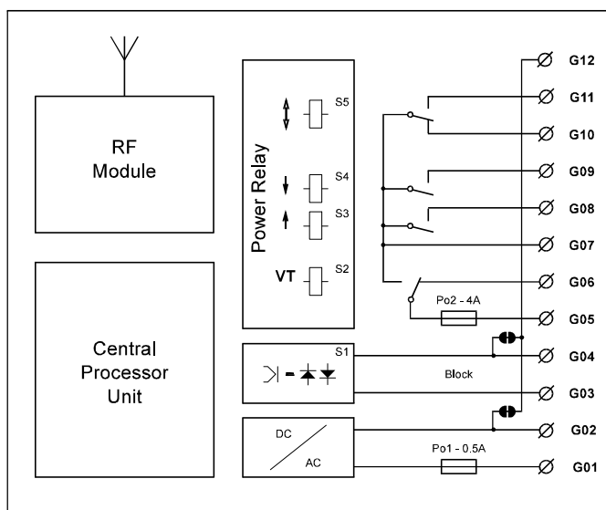
Obr.4: Liniové schéma řídicího bloku
